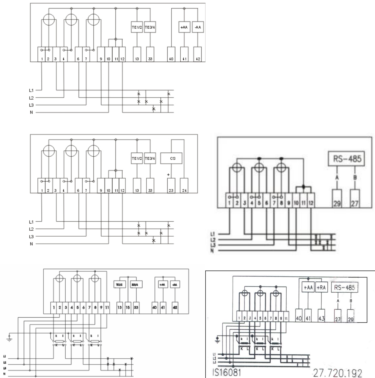
Joon. 10 – Lülituskeemid
